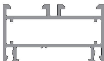
6269 0,670 Kg/m
