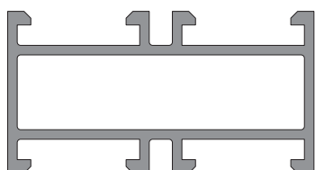
6270 0,651 Kg/m
