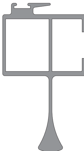
6904 1.088 Kg/m
