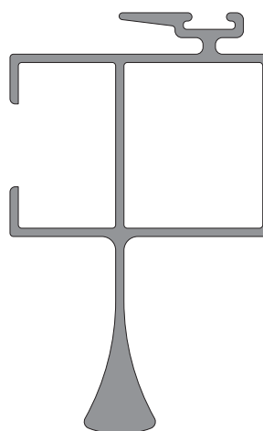
6208 0,813 Kg/m
