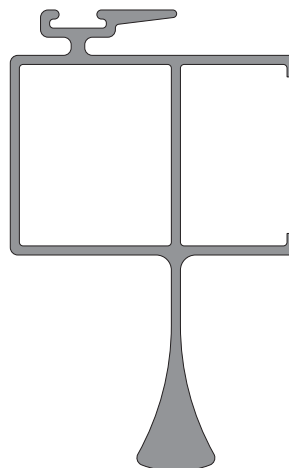
6251 0,783 Kg/m
