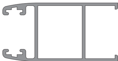
6248 0,594 Kg/m
