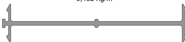
6903 0,462 Kg/m
