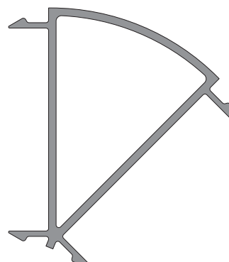
6265 0,543 Kg/m
