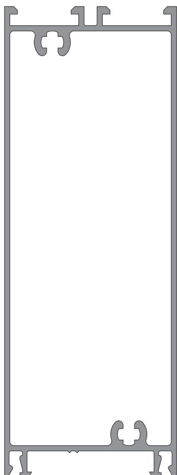
6263 1,679 Kg/m
