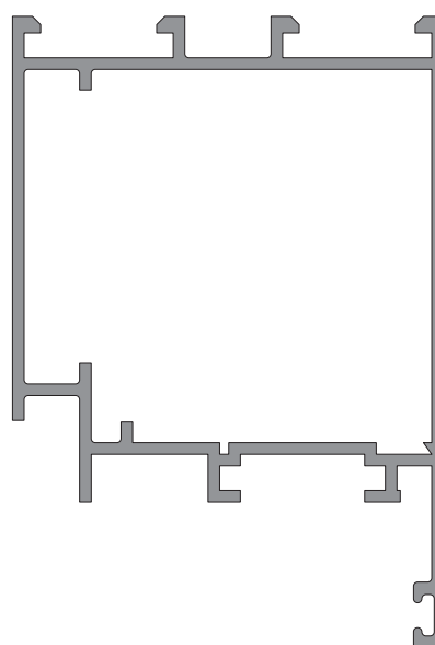
6214 1,088 Kg/m
