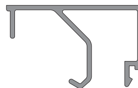
6212 0,316 Kg/m
