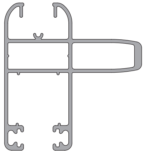
6910 1.183 kg/m
