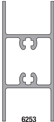
6253 0.689 kg/m
