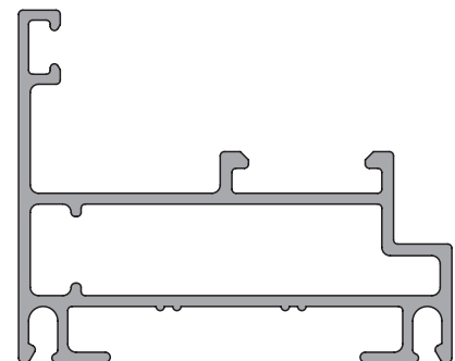
7707 0.772 kg/m
