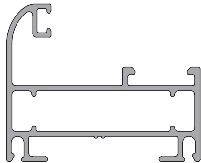
7705 0.821 kg/m
