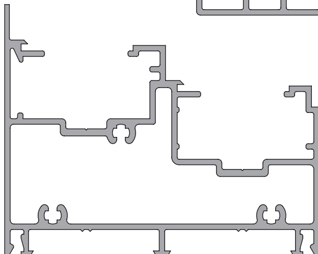
6296 1.636 kg/m
