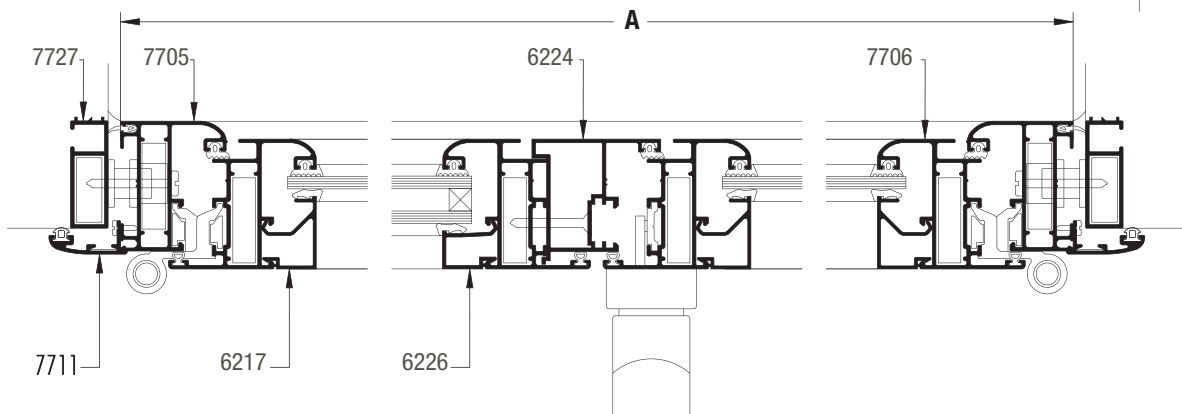
SECCION 1-5-6
