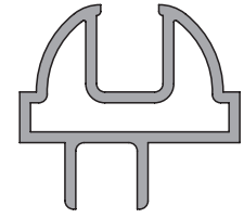
6266 0.383 kg/m
