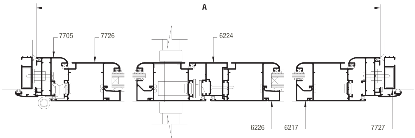
SECCION 1-2-3
