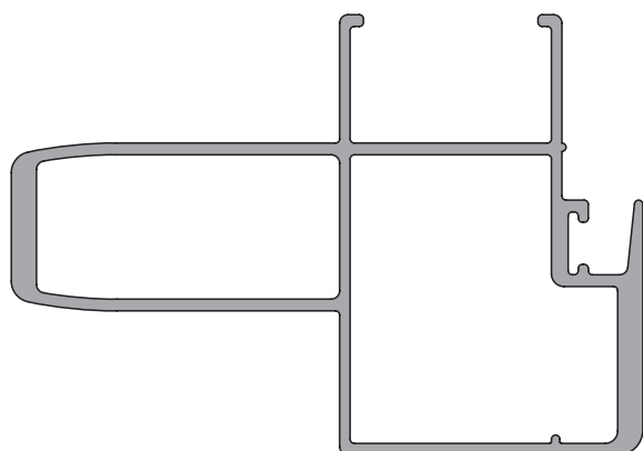
7918 1.195 kg/m
