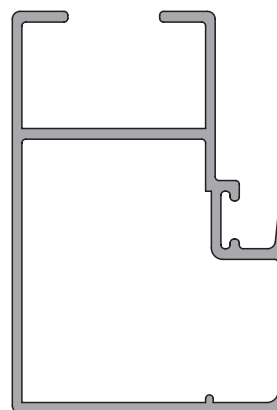
7716 0.710 kg/m
