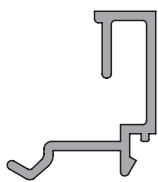
6238 0.189 kg/m
