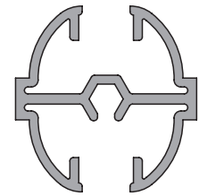
6268 0.429 kg/m
