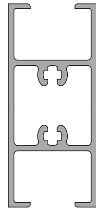
6239 0.748 kg/m
