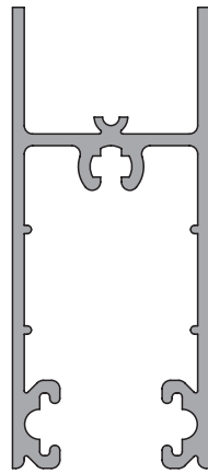
6249 0.689 kg/m
