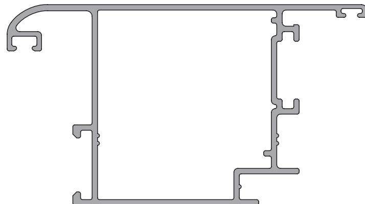
7877 1.185 kg/m
