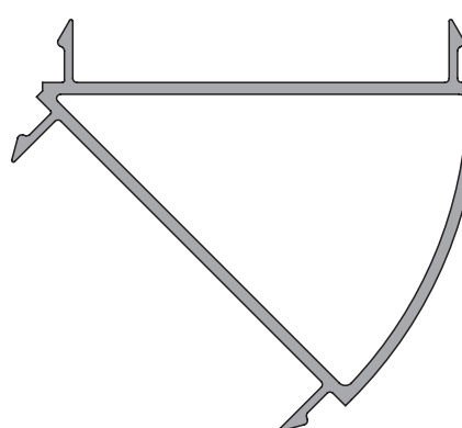
7719 0.632 kg/m
