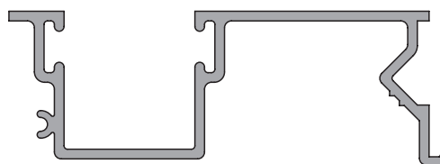
6243 0.548 kg/m
